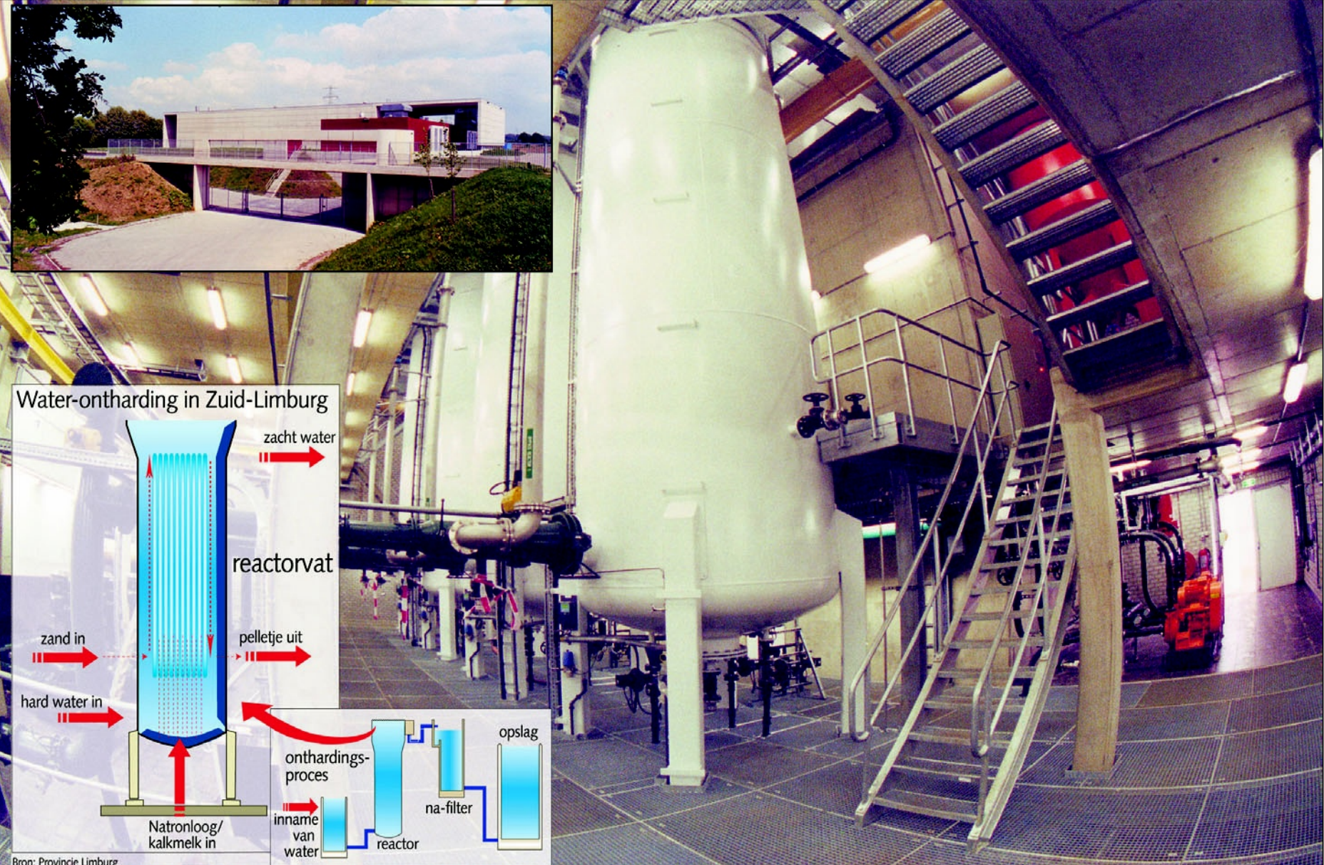
Een schematische weergave van het onthardingsproces bij WML en foto's van de onthardingsinstallatie in Amby. foto's WML
